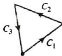
ii) C = C_1 \cup C_2 \cup C_3
