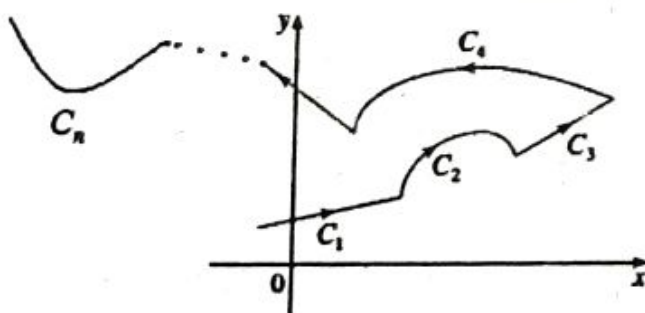
i) C = C_1 \cup C_2 \cup \dots \cup C_n
